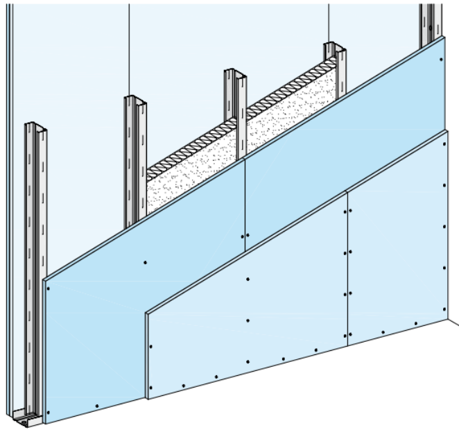
Εικόνα 8: Σύστημα με διπλή γυψοσανίδα
