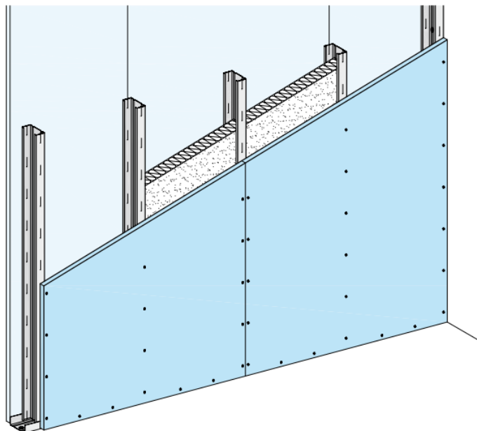
Εικόνα 7: Σύστημα με μονή γυψοσανίδα
