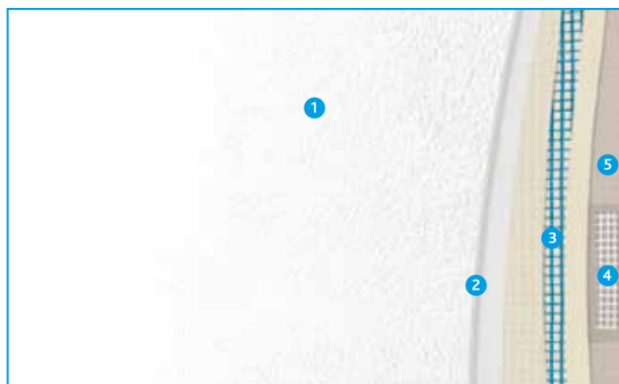
Εικόνα 5: Στρώσεις τελικής επιφάνειας τσιμεντοσανίδας.
