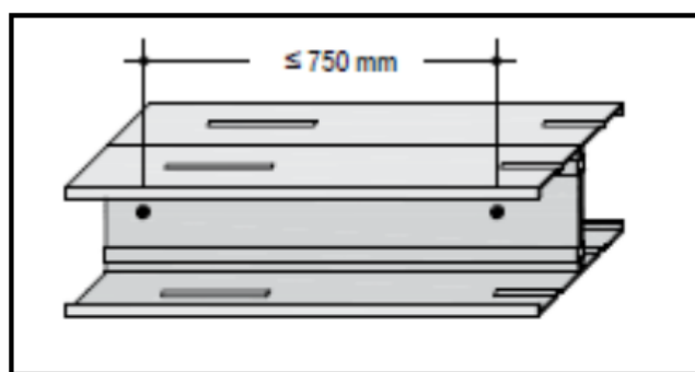
Εικόνα 4: Διπλοί ορθοστάτες τσιμεντοσανίδας.
