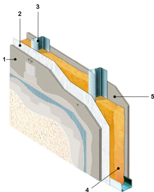
Εικόνα 3: Αξονομετρική τομή εξωτερικής τοιχοποιίας.
