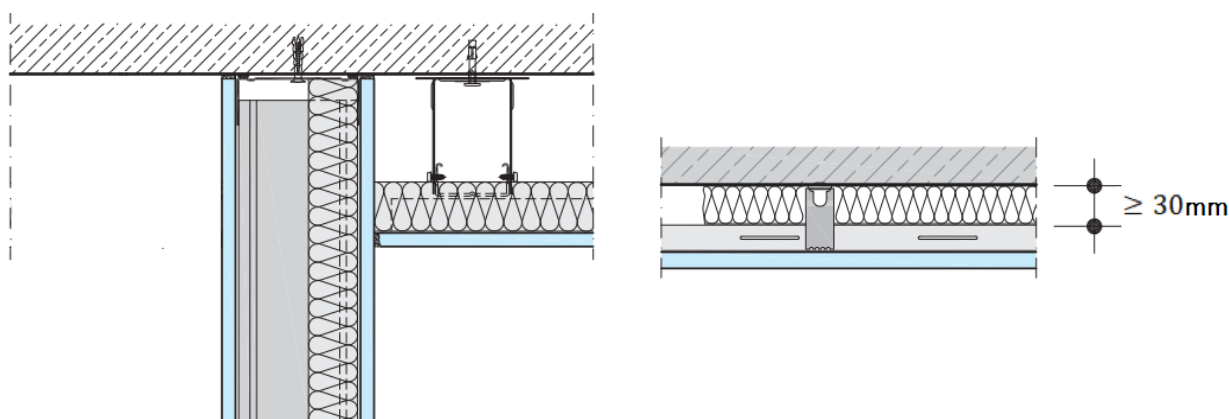
Εικόνα 9: Σύνδεση ψευδοροφής με διαχωριστικό τοίχο.
