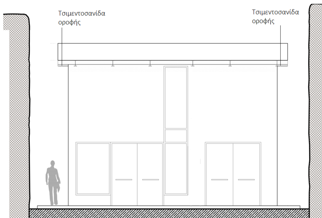
Εικόνα 6: Όψη κτιρίου με τσιμεντοσανίδα οροφής
