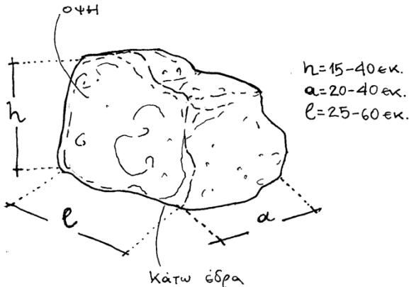
Εικόνα 5 Σκαρίφημα λίθων για την κατασκευή των παρειών
