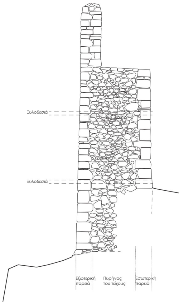
Εικόνα 3 Σκαρίφημα κατασκευαστικής τομής του τείχους
