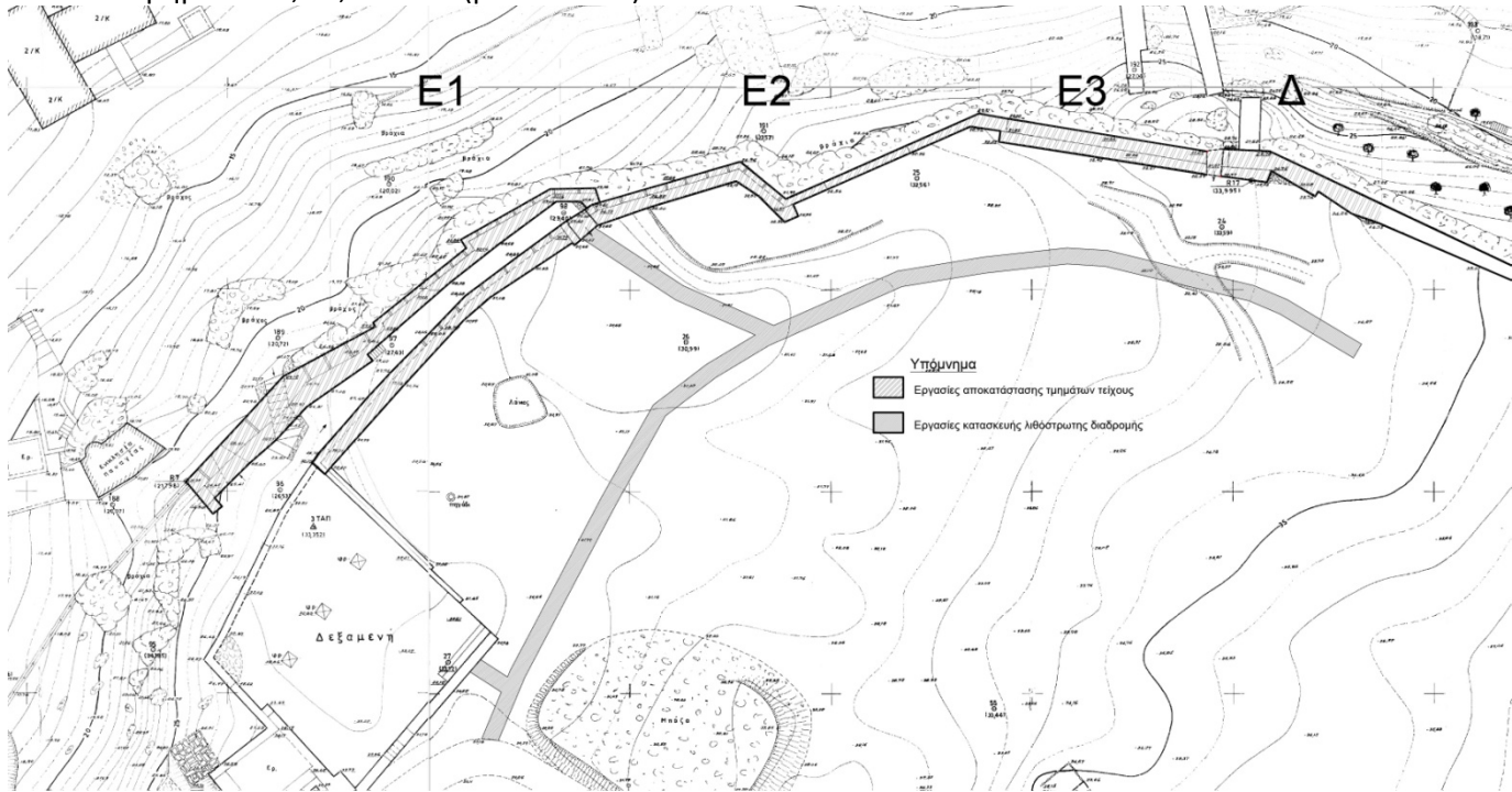
Εικόνα 1 Τοπογραφικό διάγραμμα περιοχής επέμβασης
