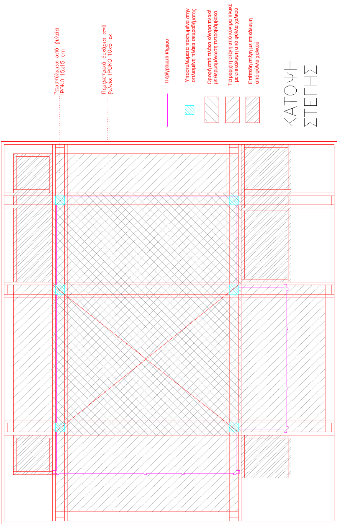
Εικόνα 11: Κάτοψη στέγης φυλακίου
