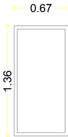
Εικόνα 8: Εξωτερικά παράθυρα φυλακίου με ανοιγόμενα και σταθερά τμήματα
