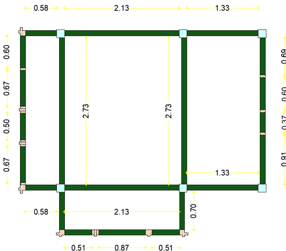
Εικόνα 5: Δοκάρια στο ύψος του ταβανιού του κτιρίου
