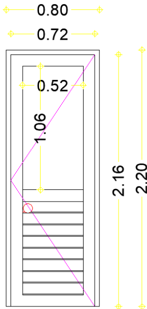
Εικόνα 9: Εξωτερική θύρα φυλακίου
