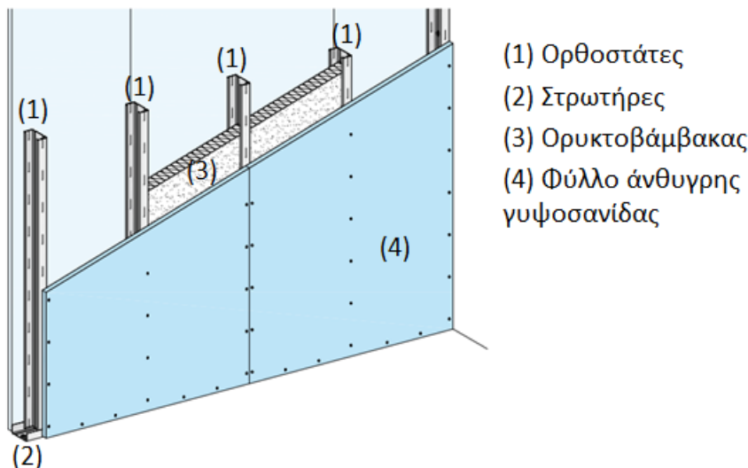
Εικόνα 12 : Σύστημα με μονή γυψοσανίδα εκατέρωθεν του μεταλλικού σκελετού
