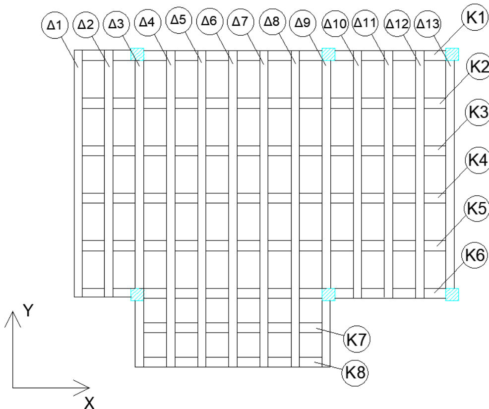
Εικόνα 4: Κάτοψη θεμελίωσης με υποστυλώματα και εσχάρα δοκαριών.
