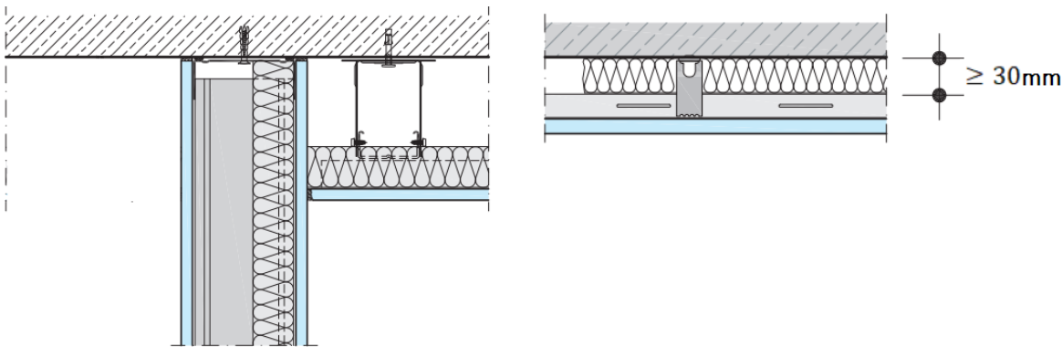
Εικόνα 13: Σύνδεση ψευδοροφής με διαχωριστικό τοίχο.
