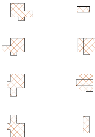
Εικόνα 6: Διαφορετικές διατομές ξύλινων υποστυλωμάτων τοιχοποιίας φυλακίου
