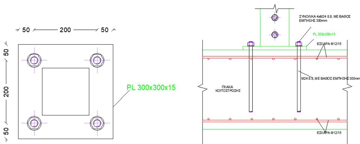
Εικόνα 3: Λεπτομέρειες έδρασης υποστυλωμάτων
