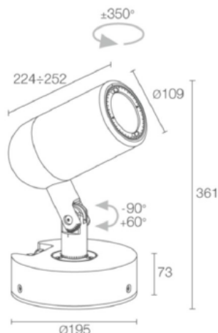
Εικόνα 4: Προβολέας LED που θα τοποθετηθεί εξωτερικά των τειχών
