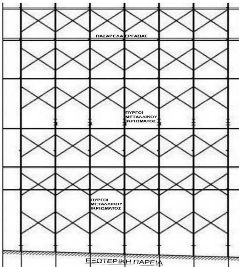
Σχέδιο 2: Ενδεικτική όψη κριωμάτων
