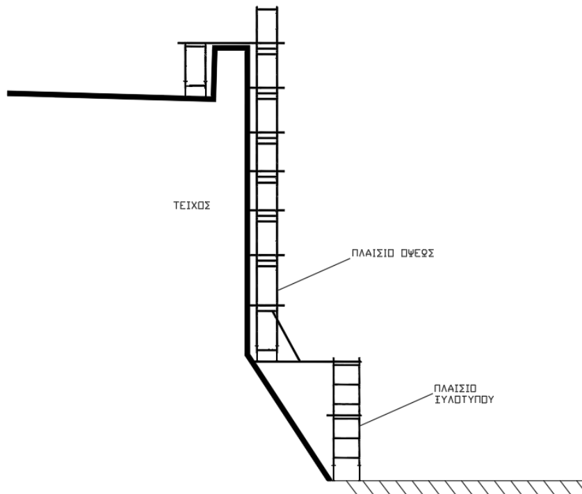
Σχέδιο 2: Ενδεικτική όψη κριωμάτων
